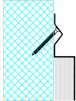
(D) (3" - 18" EJ)
